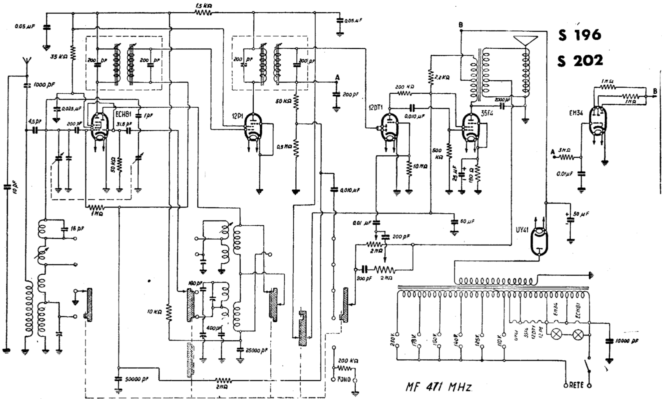
MAGNADYNE RADIO - Mod. S 196 e S 202. Onde medie suddivise e due bande allargate onde corte. Lo stadio finale è provvisto di controreazione. Potenza di uscita 3,5 watt.
